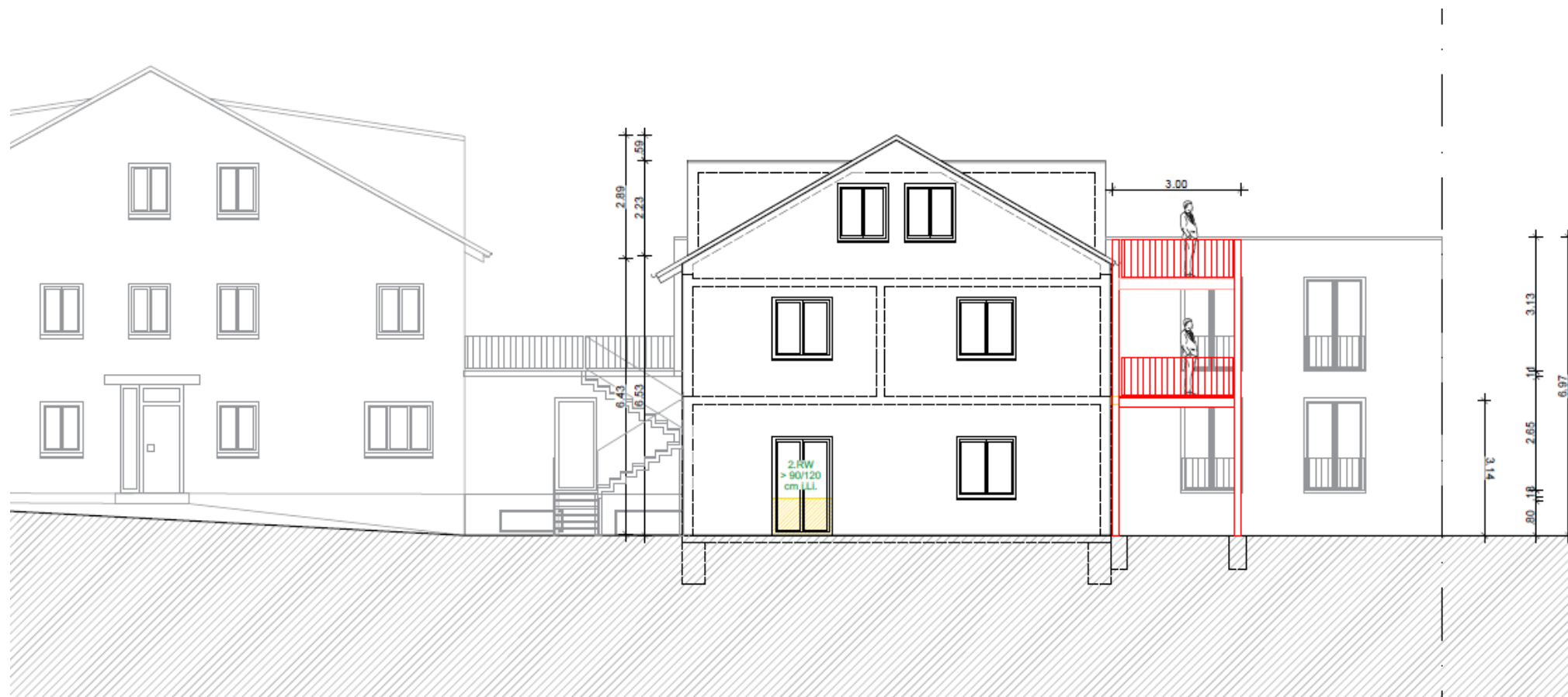
Ansicht SÜD Wohnhaus
