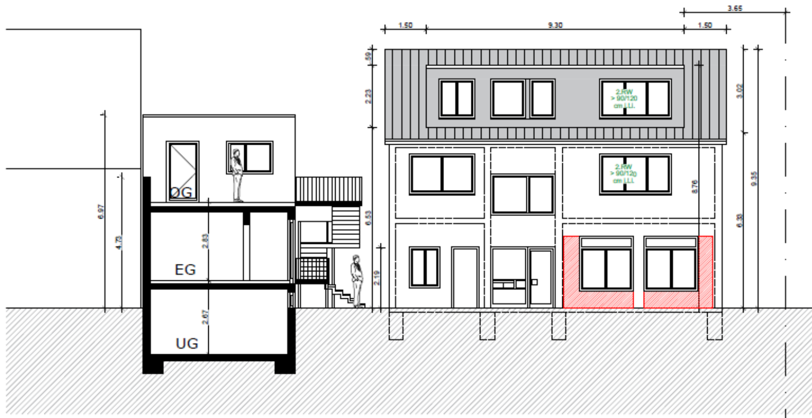
Schnitt B - B, Ansicht WEST Wohnhaus
