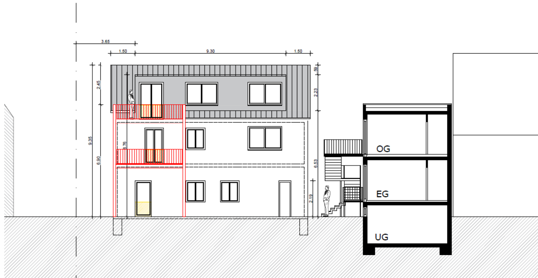
Ansicht OST Wohnhaus
