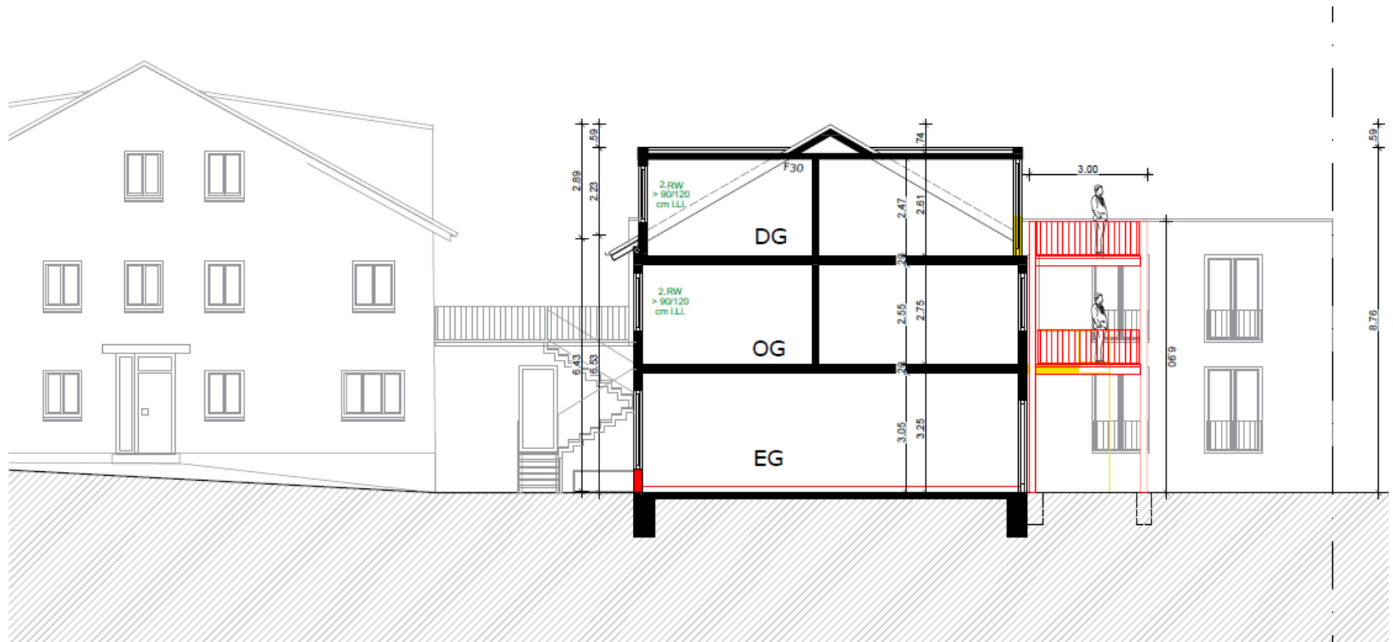
Schnitt C - C
